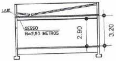
ALTURA DO GESSO SALAS E CORREDOR ESCALA..... 1/250
