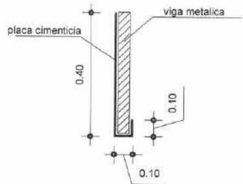
DETALHE REVESTIMENTO DA PLACA CIMENTICIA SEM ESCALA
