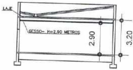
CORTE - ALTURA DO GESSO ESCALA.....1/200
